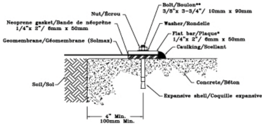
Concrete attachment detail Détail d'ancrage sur béton
