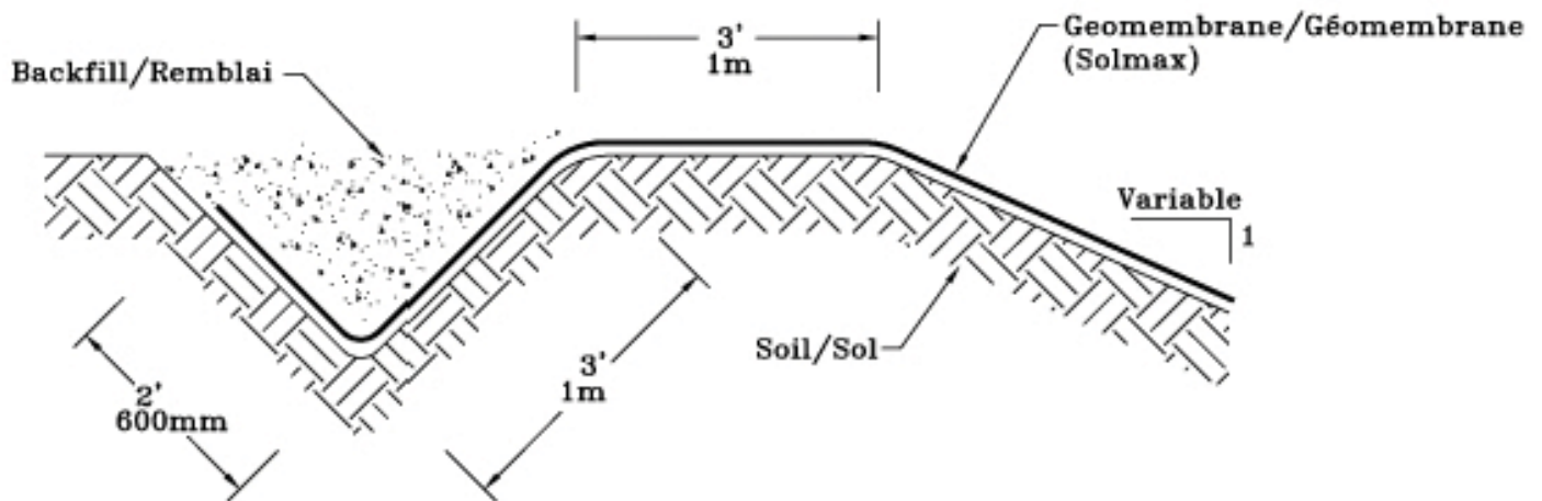
" V" anchor trench/Tranché d'ancrage en "V"
